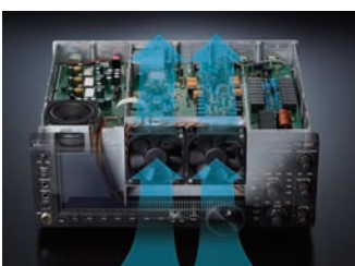
Die beiden Ventilatoren liegen hinter der Frontplatte
